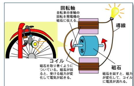
電気が起きるしくみ
